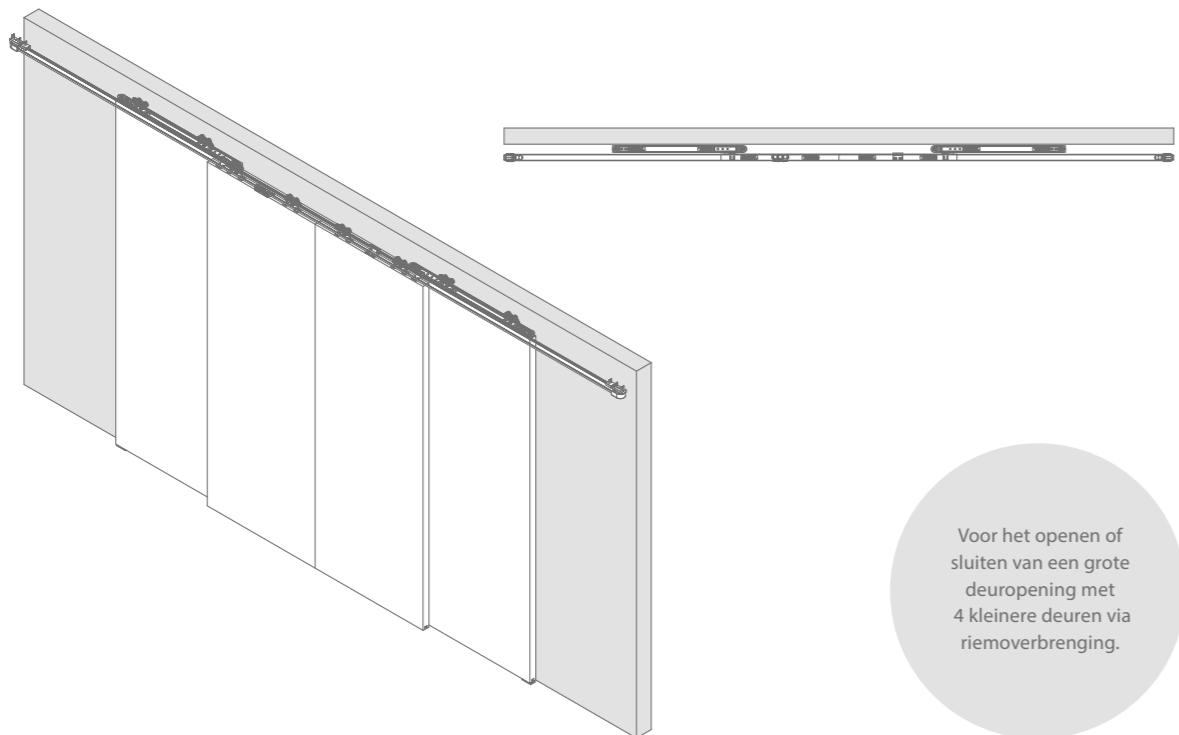
perspectief gesloten
