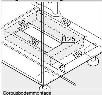
Corpusbodemmontage
